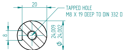
Przekrój A-A 1:1
